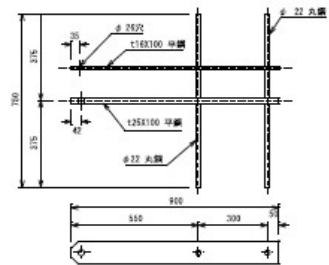
基礎Bアンカーバー S=1/10
