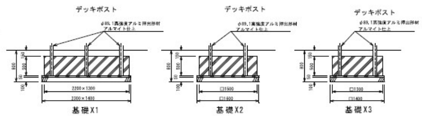
基礎詳細図 S=1/30
