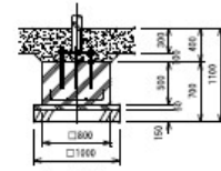
基礎A S=1/30
