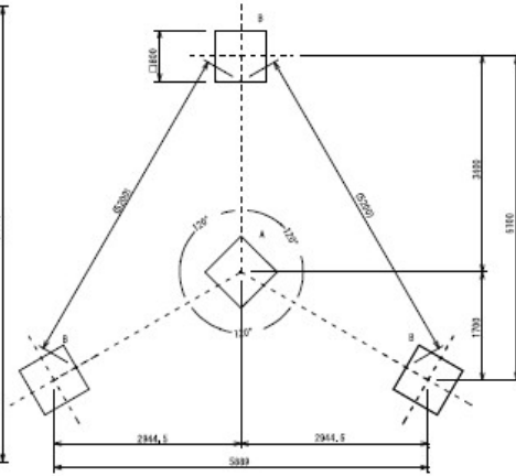
基礎状図 S=1/40
