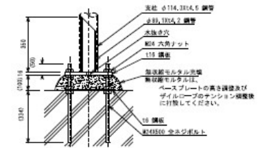
基礎Aベースプレート S=1/10
