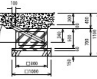
基礎B S=1/30
