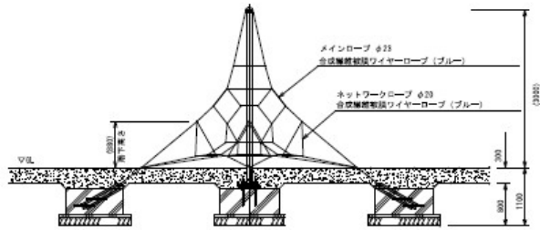
外観図 S=1/40
